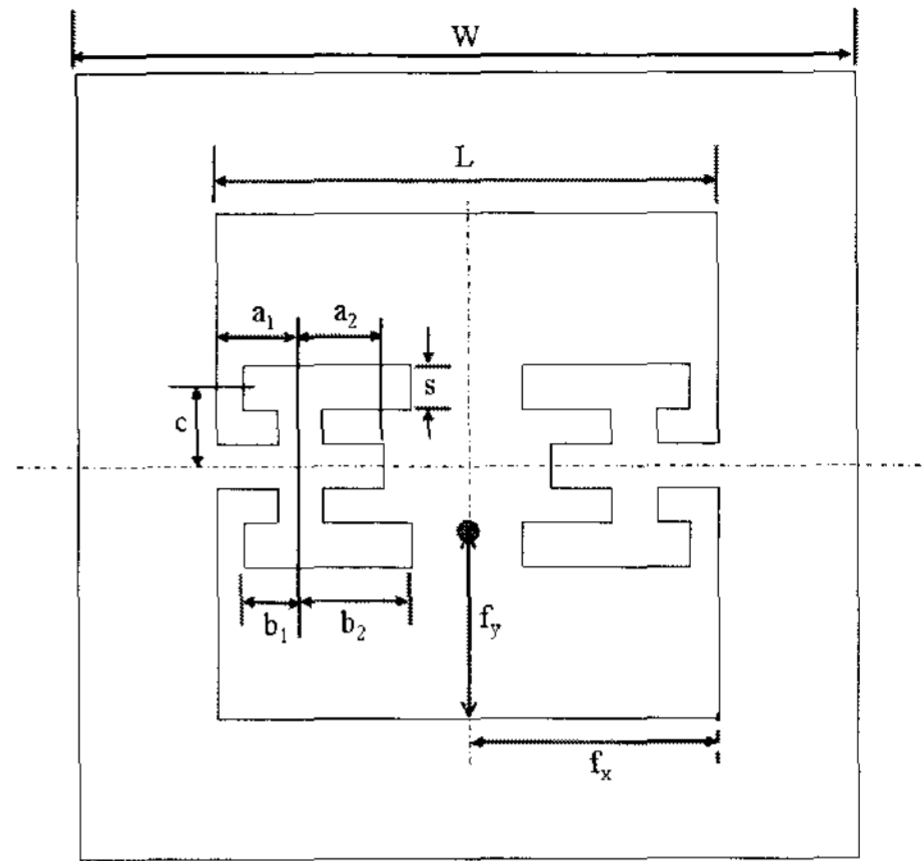
그림 3. 설계된 슬롯 안테나의 패치구조 Fig. 3 Patch structure of the slot antenna
