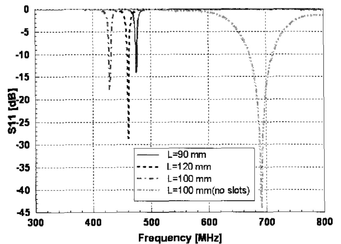
그림 4. 패치 크기에 따른 공진 주파수의 변화 Fig. 4 Variation of resonant frequencies according to the patch size
