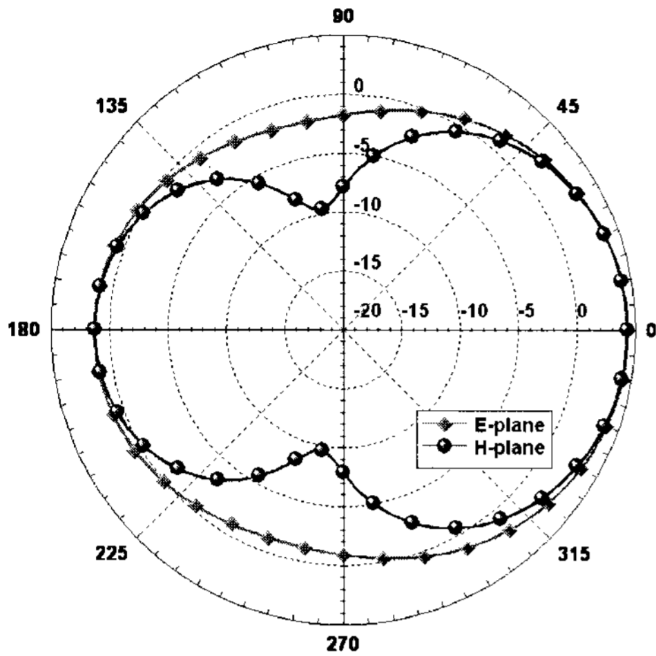
그림 5. 429 MHz에서 복사패턴 시뮬레이션 결과 Fig. Simulated radiation pattern at 429 MHz
