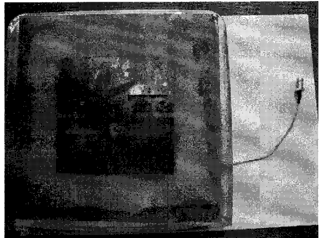
그림 7. 슬롯 장하 UHF 안테나의 제작 사진 (중심주파수: 425.6MHz, 크기: 180×180mm) Fig. 7 Picture of fabricated patch antenna
