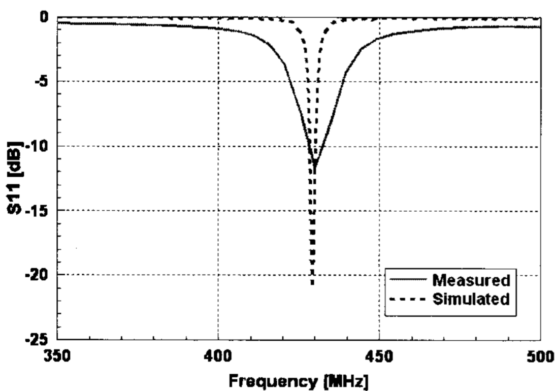
그림 6. 반사손실(S11)의 시뮬레이션과 측정결과 비교 (패치크기 L=100mm, 코팅 후 측정)
