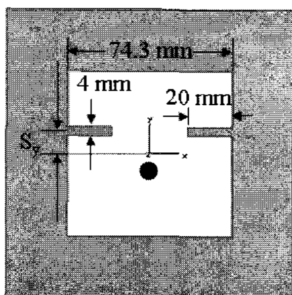
그림 1. 이중 슬롯이 장하된 패치 안테나 Fig. 1 Patch antenna loaded with double slots
