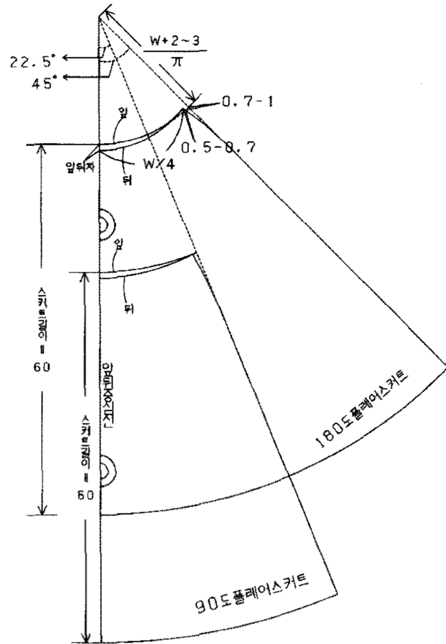
〈그림 5〉 원호를 이용한 플레어 스커트 패턴.
