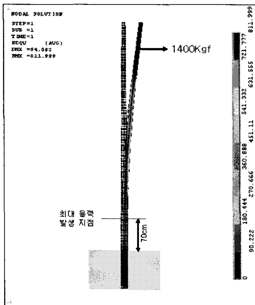
[그림 4] 16m 전신주의 파괴 하중 결과 [Fig. 4] Result of Breakdown Load for 16m Electric Pole
