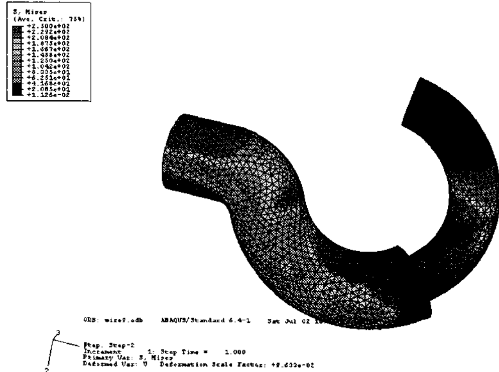
[그림 7] 유한 요소 해석 [Fig. 7] Analysis of Finite Element Method
