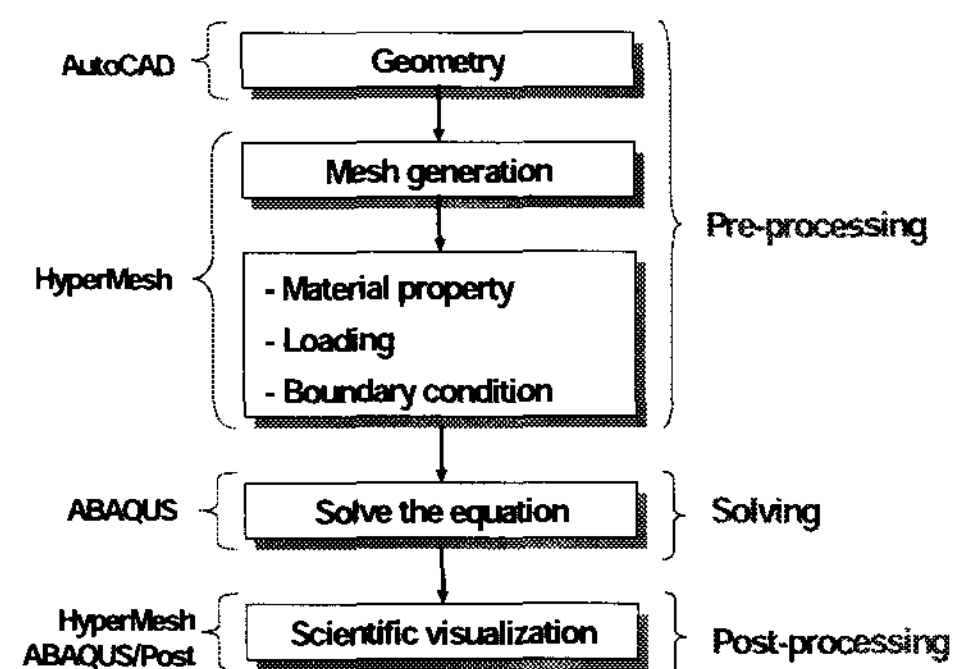
[그림 1] 유한 요소 해석 절차
