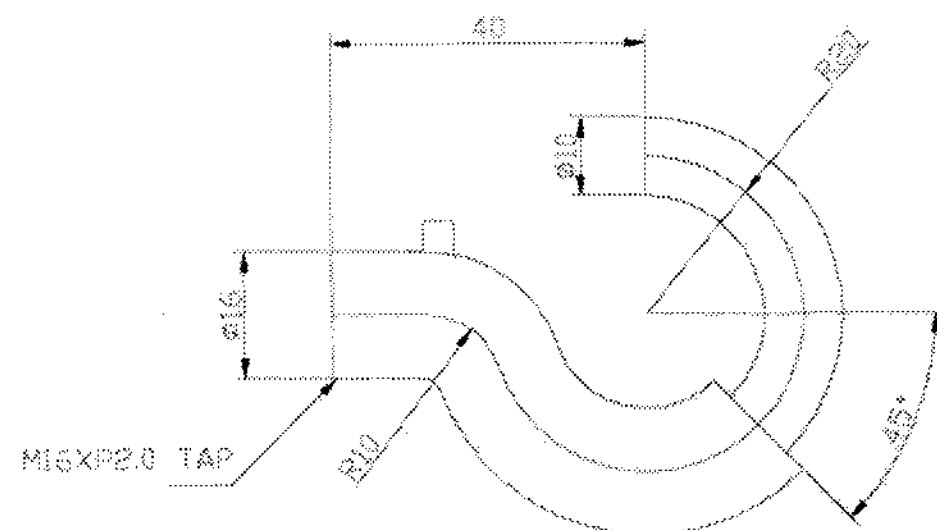
[그림 6] 전주 및 광통신선 보호용 기구 개략도 [Fig. 6] Outline of Tool for Protection of Electric Pole and Optical Communication line
