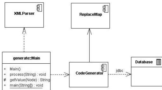
(그림 9) SQL래퍼 빌드틀의 컴포넌트 연관도
