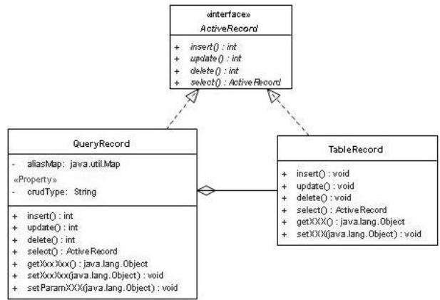
(그림 7) SQL래퍼 상위 클래스
