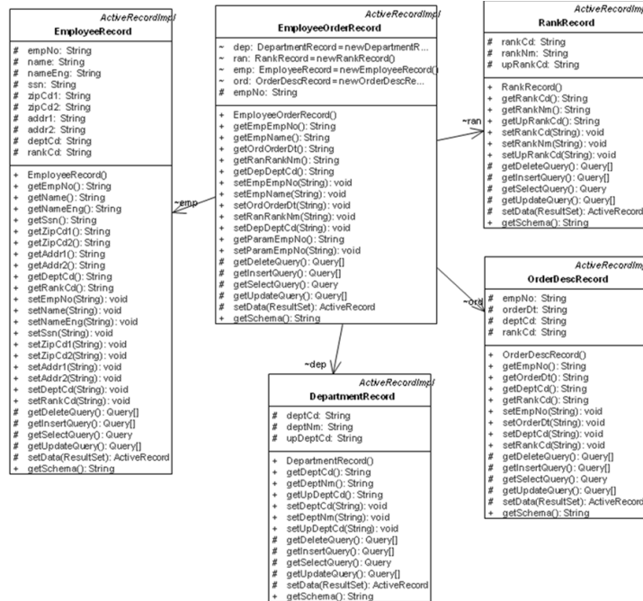
(그림 8) 빌드틀로 생성된 SQL래퍼
