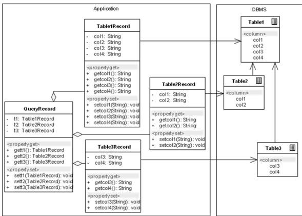
(그림 6) SQL래퍼의 ActiveRecord
