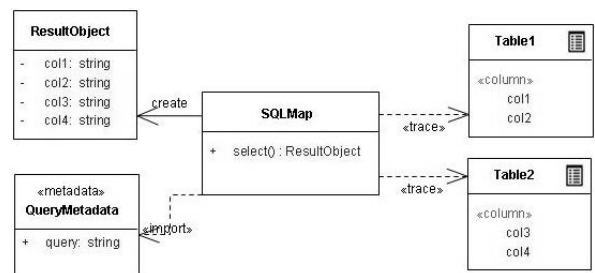
(그림 2) SQL Mapping Architecture[6]
