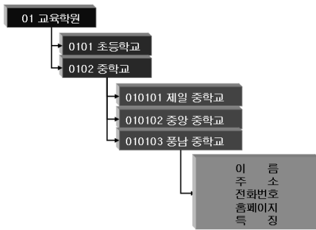
(그림 3) 3-Layer POI의 실례
