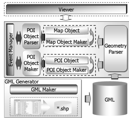
(그림 4) GVP의 전체 시스템 구조
