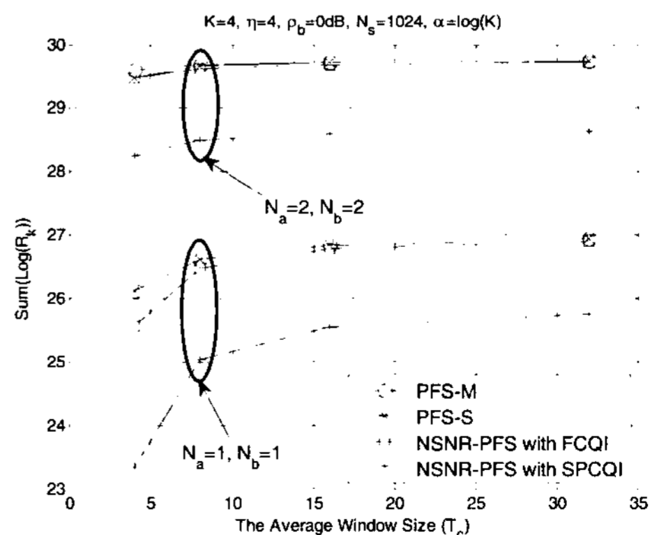
그림 1. T_c 에 따른 각 스케줄링의 비례적 공정성
