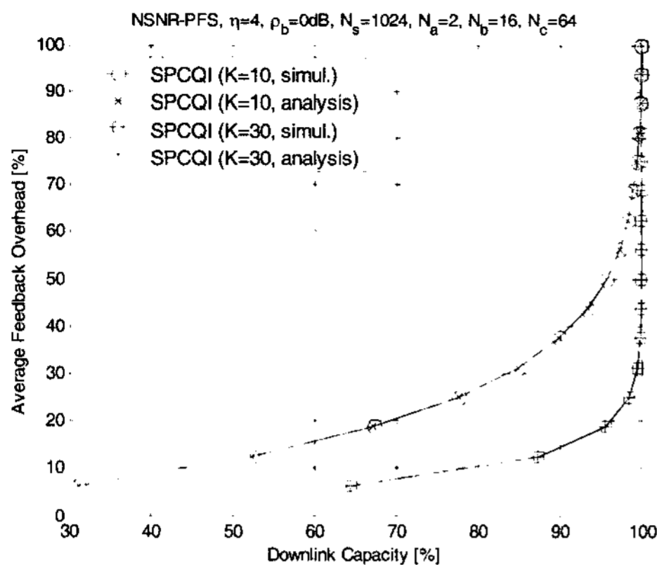
그림 2. SPCQI 기법의 하향 링크 채널 용량에 따라 요구되는 평균 채널량
