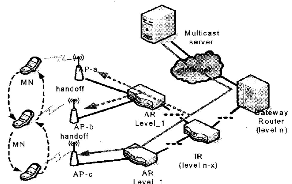
그림 4-1. 시뮬레이션을 위한 네트워크 구성
