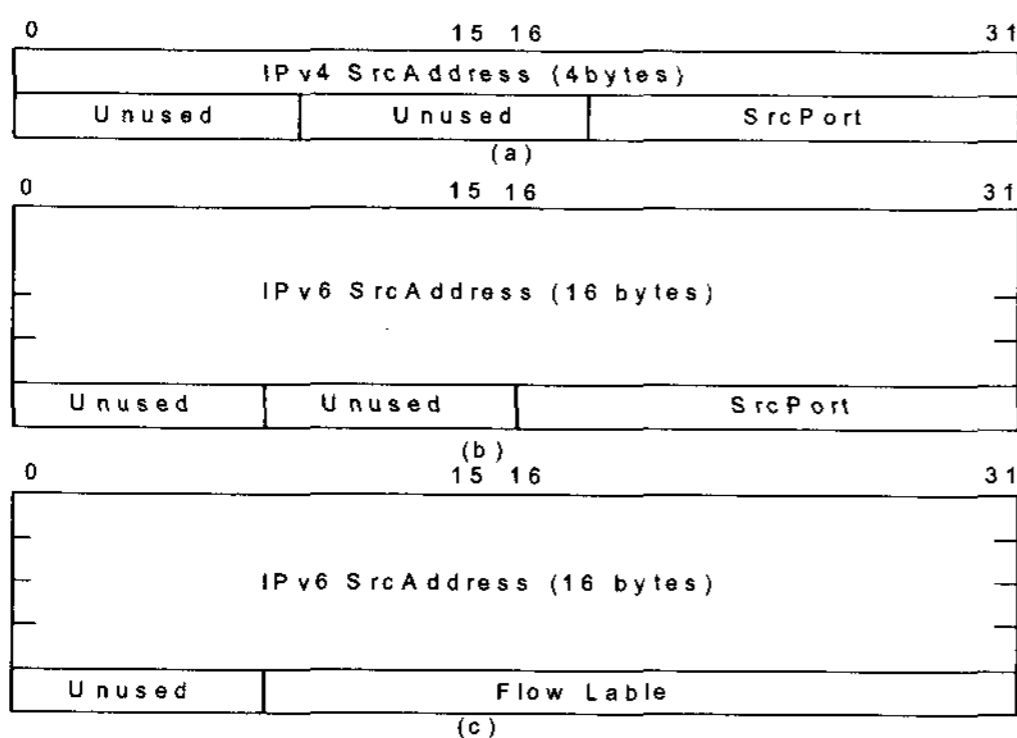
그림 3-3. filter spec의 field 형식
