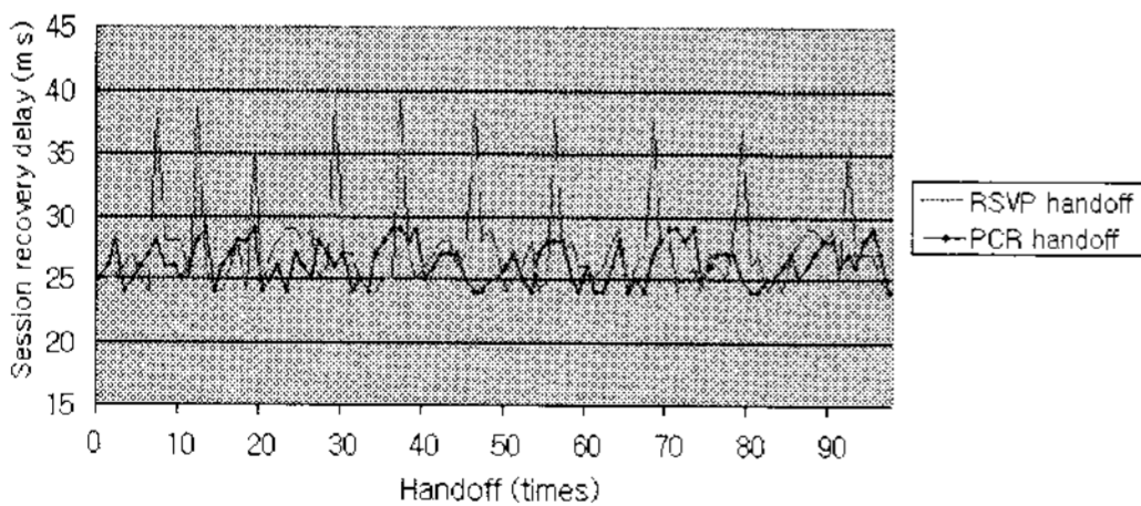
그림 4-2. Handoff 발생에 따른 경로설정 시간 변화
