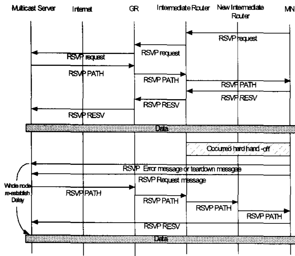
그림 3-1. Micro-mobility 네트워크의 RSVP 지원 문제점
