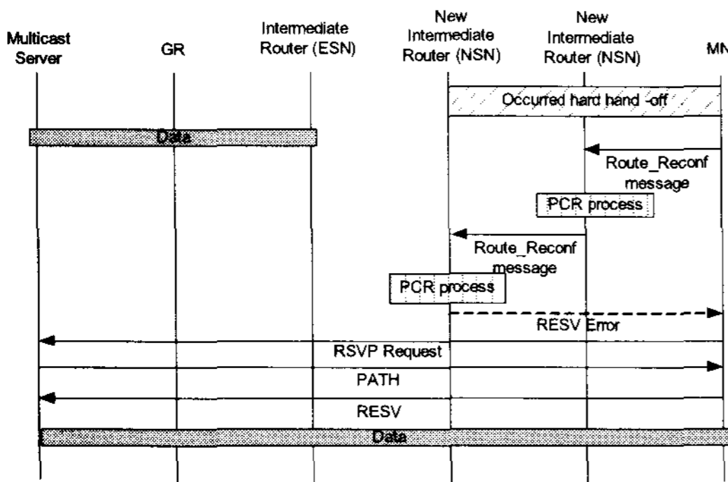
그림 3-6. PCR 알고리즘 실패시 재 설정 과정
