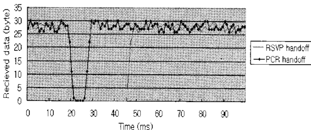
그림 4-3. handoff 이후 데이터수신 간격 비교
