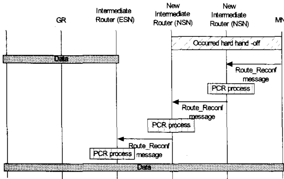
그림 3-5. PCR 알고리즘을 사용한 경로 재설정 과정
