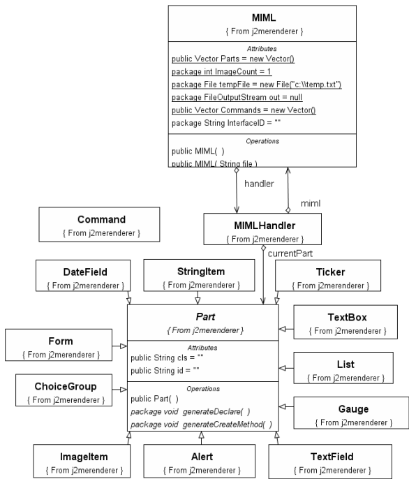
(그림 7) J2MERenderer의 클래스 구조
