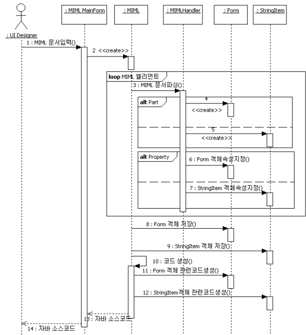
(그림 8) J2ME Renderer 코드생성과정
