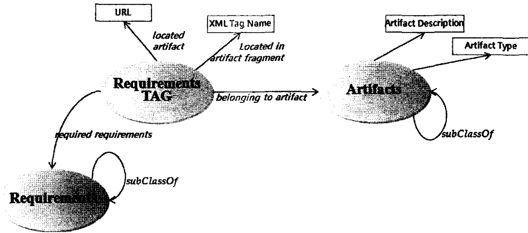
그림 2 요구사항 온톨로지를 이용한 시맨틱 태그의 표현 모델
