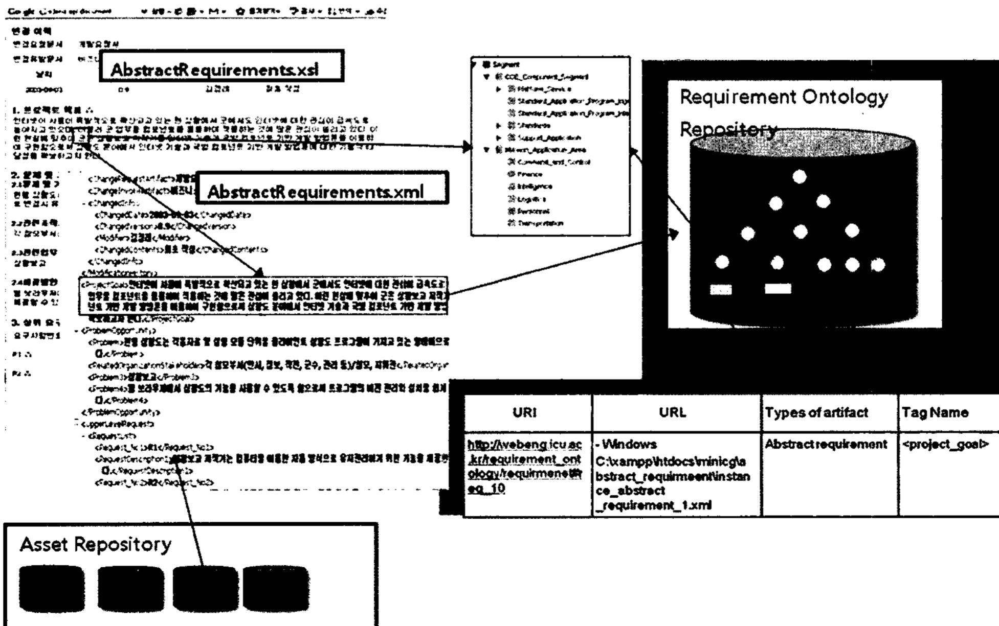
그림 5 산출물의 시맨틱 태깅 과정
