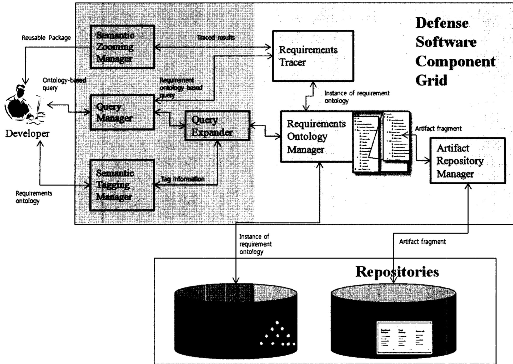
그림 1 시맨틱 태깅 기반 산출물 재사용을 위한 요구사항 추적기의 구조
