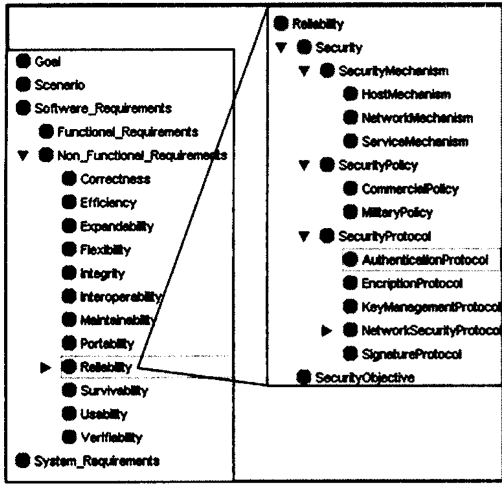
그림 4 비기능적 요구사항 온톨로지
