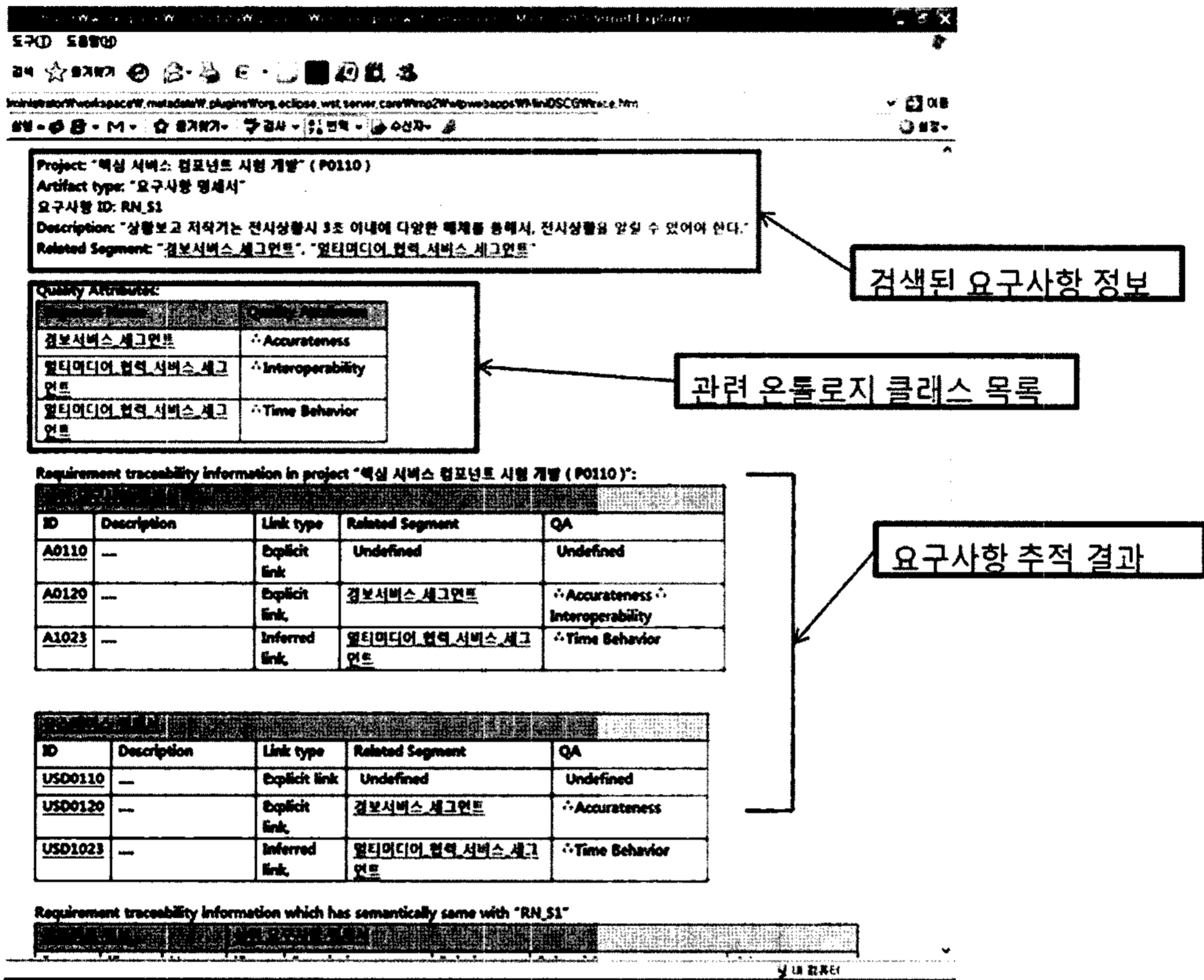
그림 7 검색된 산출물에 대한 요구사항 추적 결과
