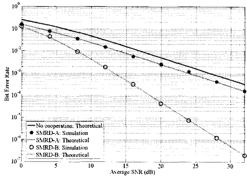
그림 7. DF에서 S와 R_1, R_2 사이의 채널이 이상적인 경우에 두 심볼의 평균에 대한 BER 성능 비교
