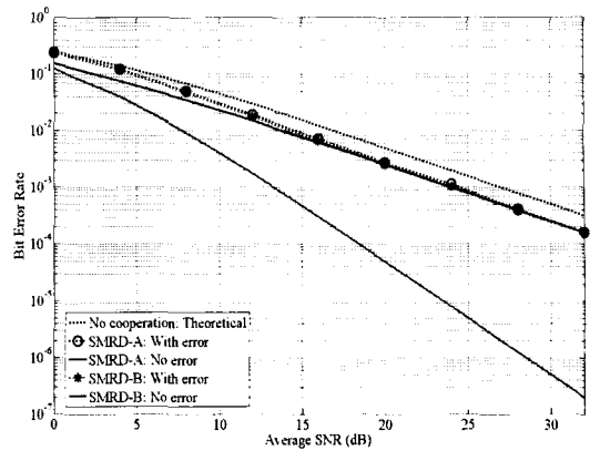
그림 8. DF에서 S 와 R_1, R_2 사이의 채널이 이상적인 경우와 이상적이지 않을 경우에 대한 BER 성능 비교
