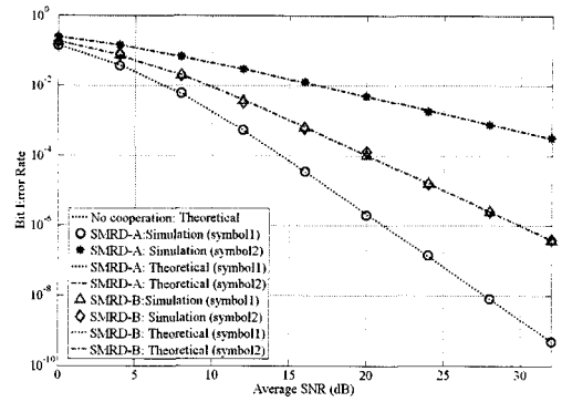
그림 5. AF에서 각 심볼에 대한 BER 성능 비교
