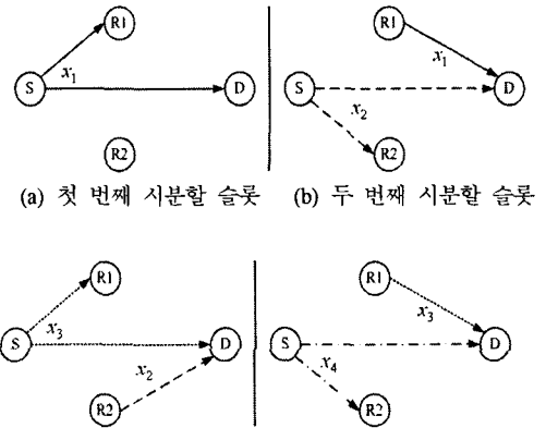
(c) 세 번째 시분할 슬롯 (d) 네 번째 시분할 슬롯 그림 3. SMRD-B 전송 프로토콜의 동작 과정
