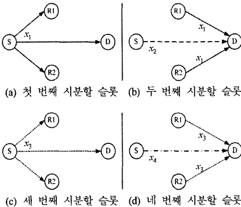
그림 2. SMRD-A 전송 프로토콜의 동작 과정
