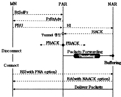
그림 1. FMIPv6의 핸드오버 처리 과정
