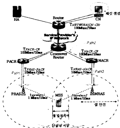
그림 3. 시뮬레이션 시스템 모델
