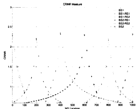
(b) 단말의 이동상황에 따른 CRINR의 변화
