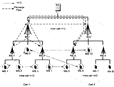
그림 1. 다중 홉 릴레이시스템에서의 핸드오버
