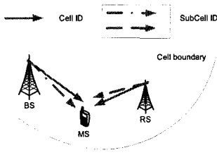
그림 4. 계층적 프리앰블을 적용한 릴레이시스템
