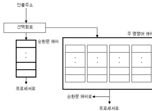
그림 2 제안하는 저전력 명령어 캐쉬 구조 Fig. 2. Proposed Energy-aware Instruction Cache
