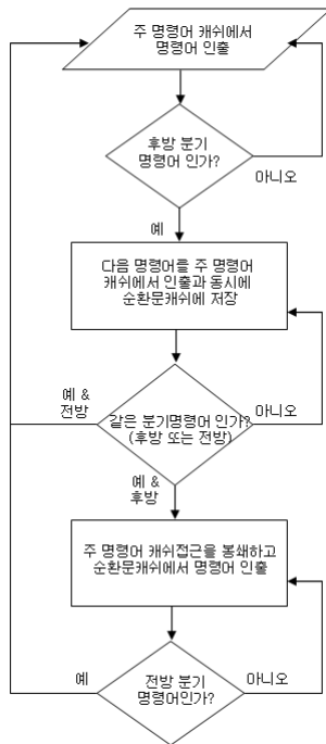
그림 3. 제안하는 저전력 명령어 캐쉬의 제어 흐름도 Fig. 3. Control Flow for the Proposed Instruction Cache
