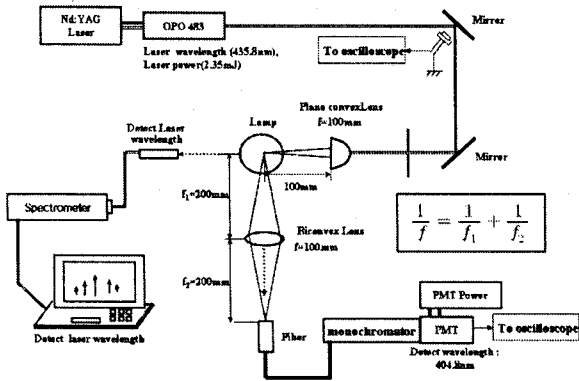
그림 4 레이저 유기 형광법 실험장치 개략도 Fig. 4 Schematic diagram of laser induced fluorescence
