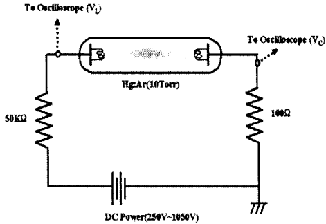
그림 3 방전 램프의 실험장치 개략도 Fig. 3 Schematic diagram of discharge lamp
