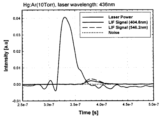
그림 5 LIF 형광신호 측정 Fig. 5 Measurement of LIF fluorescence signal
