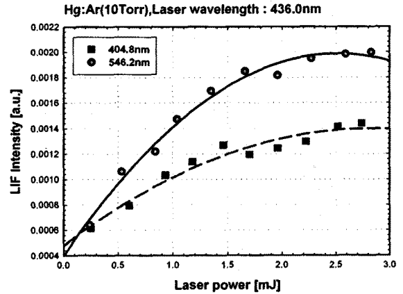
그림 8 인가 레이저 전력에 따른 LIF 형광신호 측정 Fig. 8 LIF fluorescence signal measurement according to applied power to laser
