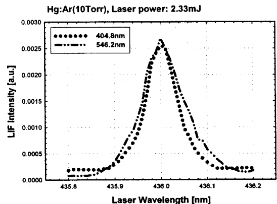
그림 6 레이저 인가 파장에 따른 LIF 형광신호 Fig. 6 LIF fluorescence signal according to laser applied wave
