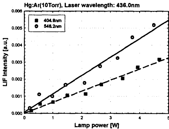
그림 7 램프 인가 전력에 따른 LIF 형광신호 Fig. 7 LIF fluorescence signal according to applied power to lamp
