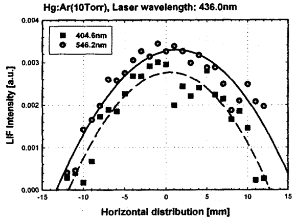
그림 9 방전램프의 수평축 플라즈마 밀도 분포 Fig. 9 Plasma density distribution
