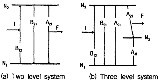
그림 2 레이저 유기 형광법의 2-level과 3-level 구조 Fig. 2 Structure of 2-level and 3-level for laser induces fluorescence
