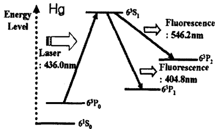
그림 1 레이저 유기 형광법의 에너지 준위 개념도 Fig. 1 Concept of energy level for laser induces fluorescence
