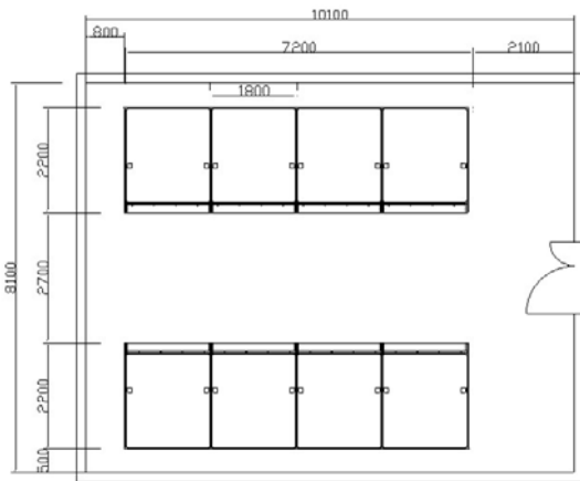
그림 1. 돈사평면
