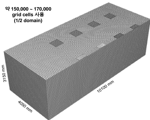
그림 5. Computational Grid
