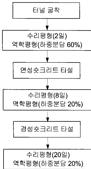
그림 2. 굴착 및 연계 해석 순서도
