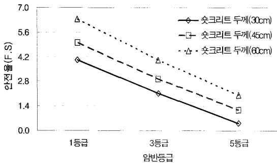
그림 14. 안전율과 암반등급의 관계(펌프 고려)
