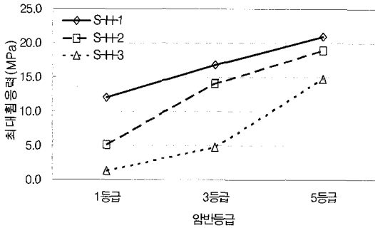
그림 12. 최대휨응력과 암반등급의 관계(shotcrete 두께 40 cm, 1층)
