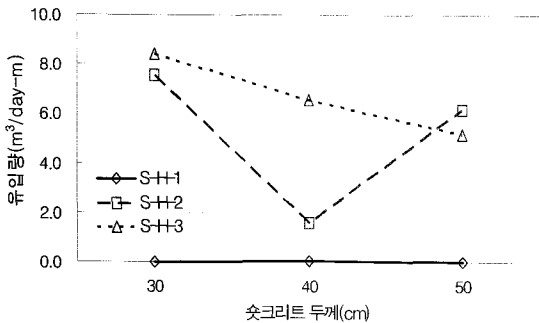
그림 9. 유입량과 숯크리트 두께의 관계(1등급, 숯크리트 모델링 3층)
