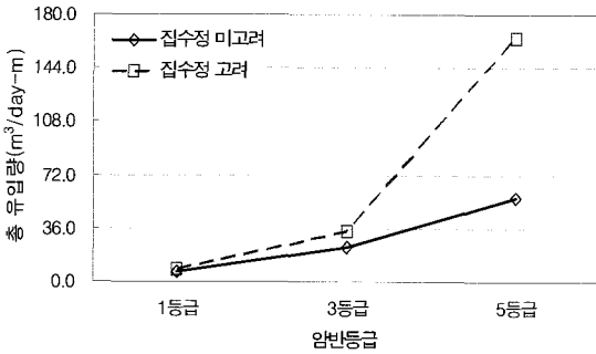
그림 18. 총 유입량과 암반등급의 관계(shotcrete 두께 45 cm)
