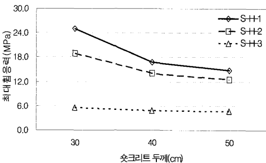
그림 13. 최대휨응력과 shotcrete 두께의 관계(3등급, 1층)
