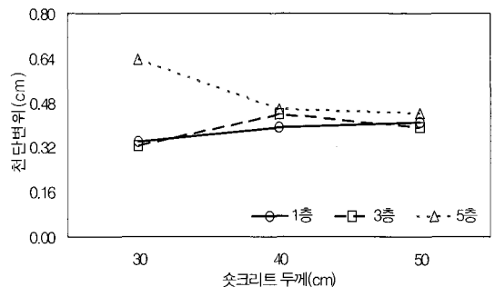
그림 11. 숯크리트 수리특성(S-H-3)의 숯크리트 두께와 천단 변위(3등급)의 관계
