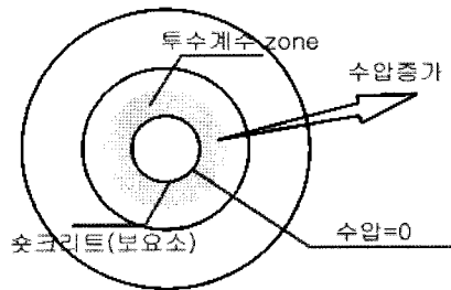
그림 3. 슛크리트 지보재 모델링(보요소)
