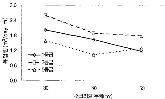
그림 10. 유입량과 숯크리트 두께의 관계(숯크리트 모델링 5층, S-H-2)
