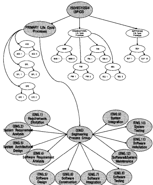
그림 5. ISO/IEC15504성숙도 및 역량 모델 표준 온톨로지 Fig 5. Standard Ontology of ISO/IEC15504
