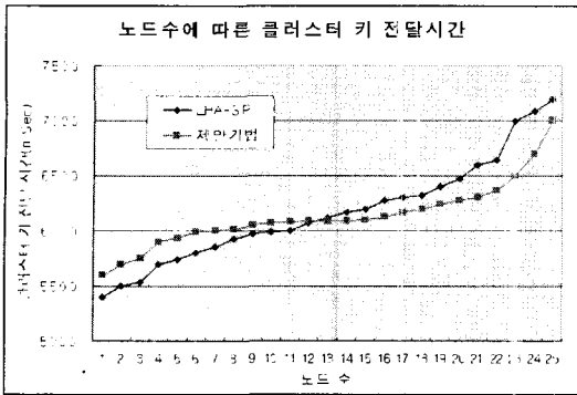
그림 6. 노드수에 따른 클러스터 키 전달시간
