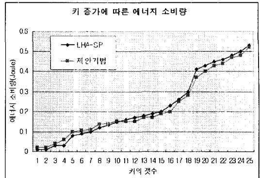
그림 8. 키 증가에 따른 에너지 소비량
