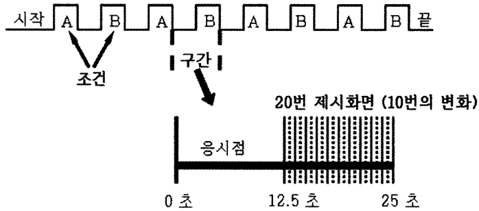
그림 2. 기능적 자기 공명 영상 촬영과 한 구간의 예시 화면
