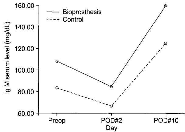
Fig. 2. Immunoglobulin M.
