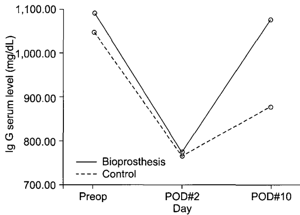
Fig. 1. Immunoglobulin G.
