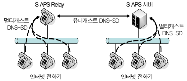
(그림 3) S-APS를 이용한 인터넷 전화 구성도
