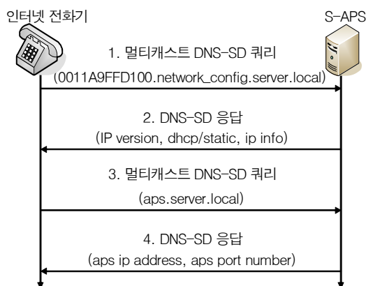
(그림 1) mDNS/DNS-SD를 이용한 S-APS 검색 및 네트워크 설정
