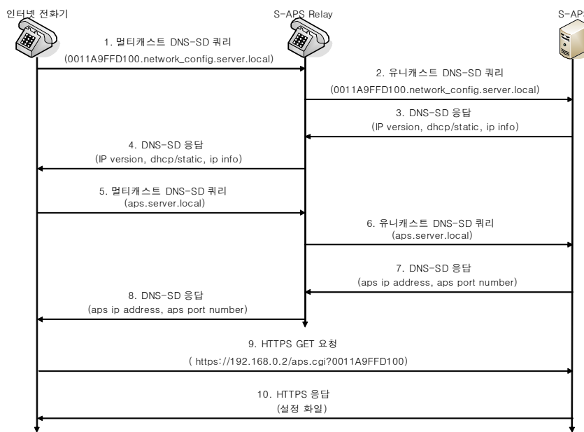
(그림 4) S-APS를 이용한 자동 프로비저닝 네트워크 흐름도
