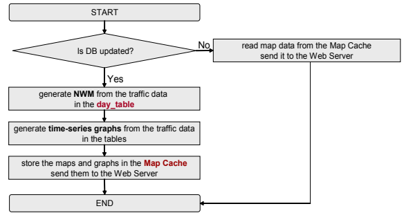
(그림 9) NWM Generator 순서도
