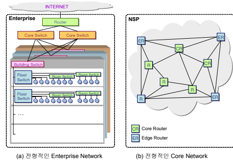
(그림 2) Enterprise 네트워크 vs. Core 네트워크
