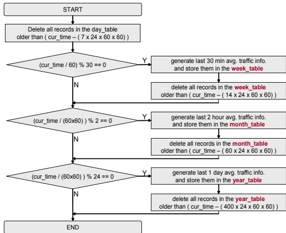
(그림 8) DB Manager 순서도
