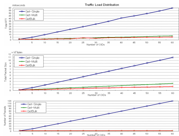
(그림 7) SNMP 메시지의 성능 비교
