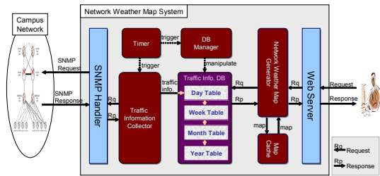
(그림 4) NWM 시스템 전체 구조
