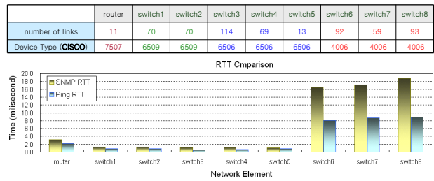
(그림 6) 캠퍼스 NWM에 사용된 네트워크 장비
