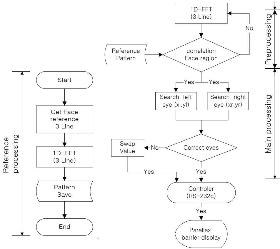
그림 15. 시점추적 흐름도.
