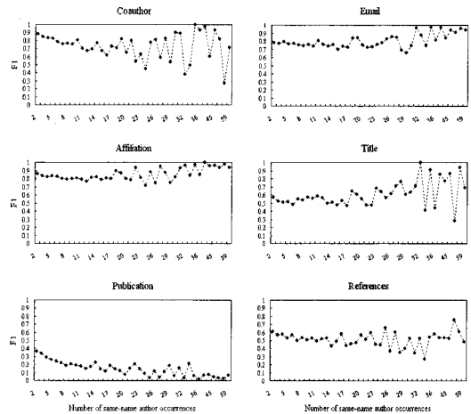
그림 1. 동명 저자 출현수와 저자 식별 성능 (저자유사도임계치=1)
