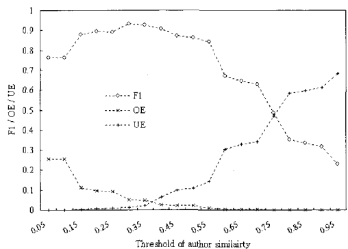
그림 2. 다중 자질 결합의 저자 식별 성능
