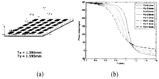
그림 2. (a) 주기적인 패치 구조, (b) 해석 결과 Fig. 2. (a) Periodic patch structures, (b) Phase results.
