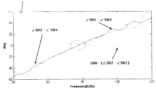
(d) Port 8 결과 (d) Results at Port 8
