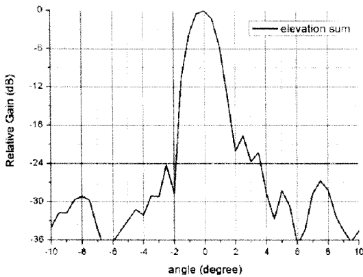
(b) 안테나의 elevation 방향의 sum 패턴 (b) Sum pattern of the antenna(elevation direction)
