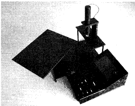
그림 5. 제작된 시스템 Fig. 5 H/W system
