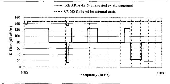
그림 6 내부 전장품에 대한 COMS RS vs Arian V RE (1GHz~10GHz) Fig. 6 The comparison between COMS RS for internal equipment and Arian V RE (1GHz~10GHz)
