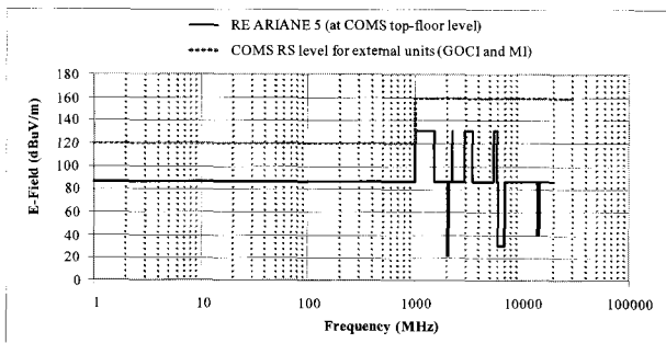
그림 7 외부 전장품에 대한 COMS RS vs Arian V RE Fig. 7 The comparison between COMS RS for external equipment and Arian V RE
