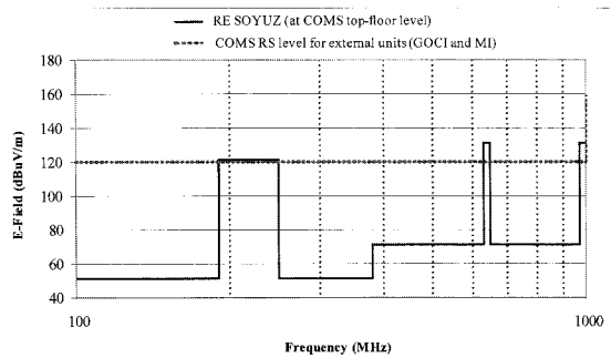
그림 13 외부 전장품에 대한 COMS RS vs SOYUZ RE (100MHz~1GHz) Fig. 13 The comparison between COMS RS for external equipment and Soyuz RE (100MHz~1GHz)
