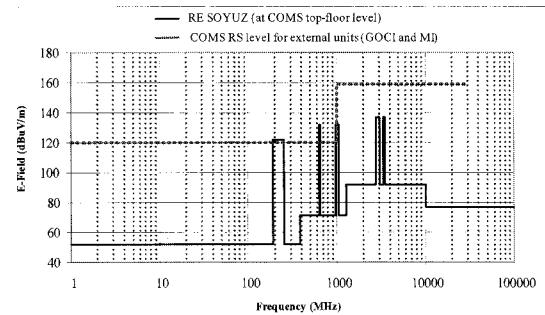
그림 12 외부 전장품에 대한 COMS RS vs Soyuz RE Fig. 12 The comparison between COMS RS for external equipment and Soyuz RE
