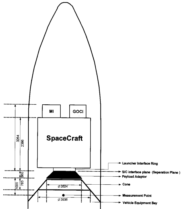
그림 3 Ariane V 페어링 내부에 탑재된 COMS 형상개략도 Fig. 3 The configuration of COMS under the Ariane V Fairing
