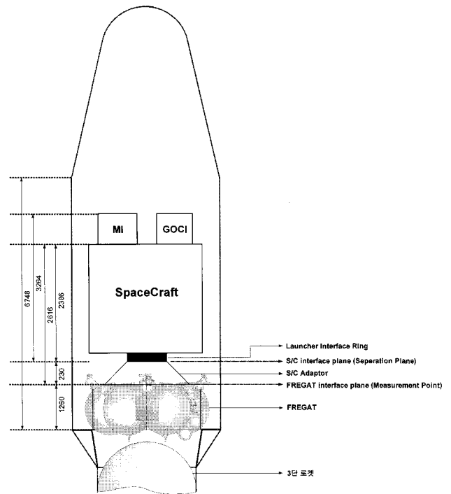
그림 11 Soyuz 페어링내부에 탑재된 COMS 형상개략도 Fig. 11 The configuration of COMS under the Soyuz Fairing
