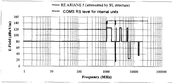
그림 5 내부 전장품에 대한 COMS RS vs Arian V RE Fig. 5 The comparison between COMS RS for internal equipment and Arian V RE
