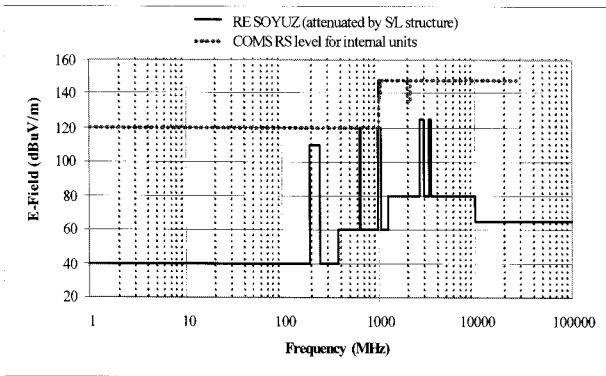
그림 9 내부 전장품에 대한 COMS RS vs Soyuz RE Fig. 9 The comparison between COMS RS for internal equipment and Soyuz RE
