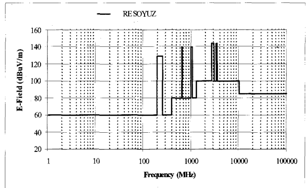
그림 8 Soyuz의 전자파 방사 수준 레벨 Fig. 8 The Radiated Emission (RE) level of Soyuz
