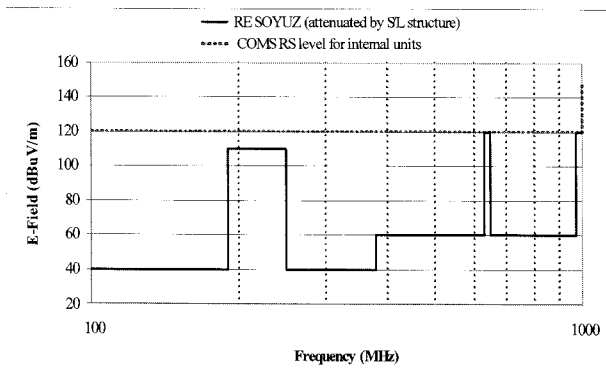
그림 10 내부 전장품에 대한 COMS RS vs Soyuz RE (100MHz~1GHz) Fig. 10 The comparison between COMS RS for internal equipment and Soyuz RE (100MHz~1GHz)
