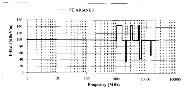
그림 4 Ariane V의 전자파 방사 수준 레벨 Fig. 4 The Radiated Emission (RE) level of Ariane V
