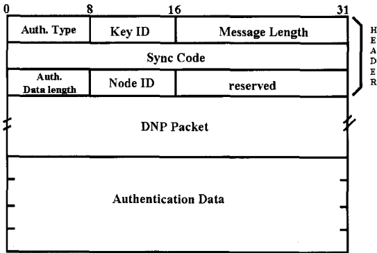
그림 3 패킷의 구성 Fig. 3 Packet format
