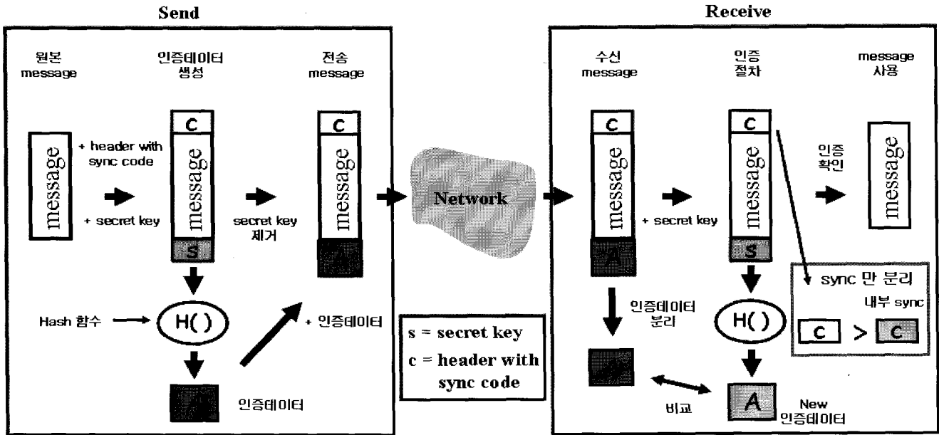
그림 2 배전자동화 시스템에 적합한 보안 알고리즘의 적용방안 Fig. 2 Applying Security Algorithms to suit to the Distribution Automation System
