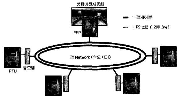
그림 1 국내 배전자동화 시스템의 통신구조 Fig. 1 Communication structure of DAS
