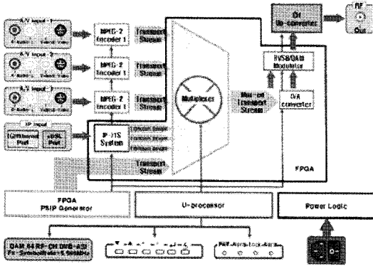
그림 2. IPMG 변조기 블록도
