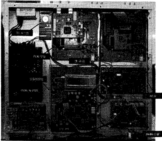
그림 15. 제작된 확장된 IPMG 내부사진
