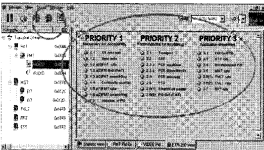
그림 20. MTS 400i로 ETR290에 준수하여 분석된 실험결과(우선순위별 에러체크)
