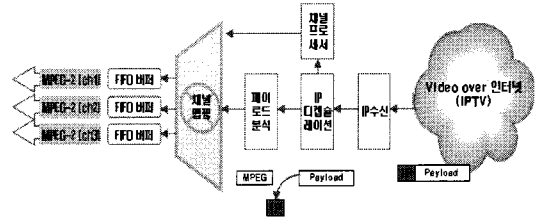
그림 7. TS 변조시스템의 동작하는 과정을 설명하는 블록도
