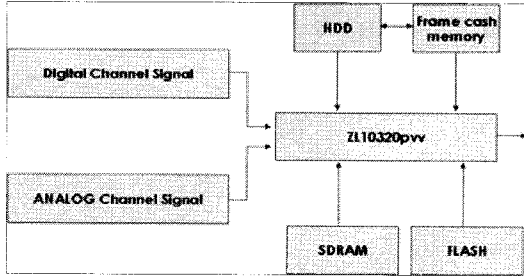
그림 12. 시차방송시스템의 동작을 설명하는 블록도
