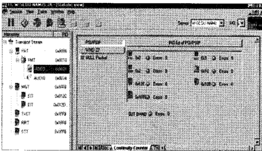
그림 19. MTS 400i로 ETR290에 준수하여 분석된 실험결과 (PSI/PSIP 에러체크)
