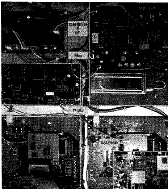
그림 3. 신호 변조 및 송출 시스템 내부사진
