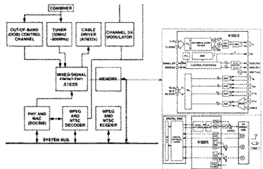
그림 10. OOB 시스템의 동작을 설명하는 블록도
