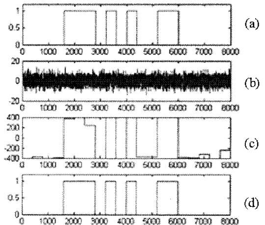
그림 8. PG=400, ONU개수=16인 경우 CDMA 번복조 과정 (a) ONU-1의 전송 ID (b) 16개 ONU 송신신호 합 (c) OLT PD에서의 CDMA 디코딩신호 (d) 복구된 ONU-1의 ID
