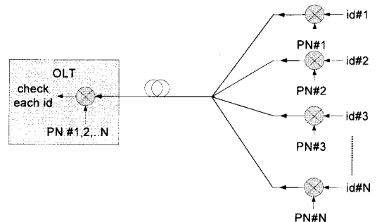
그림 3. CDMA 변조를 이용한 각 ONU의 ID 전송
