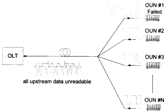
그림 1. ONU 고장 및 PON 전체 상황 통신의 중단
