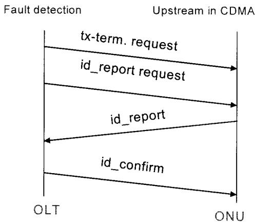
그림 2. 고장 ONU를 찾기 위한 알고리즘
