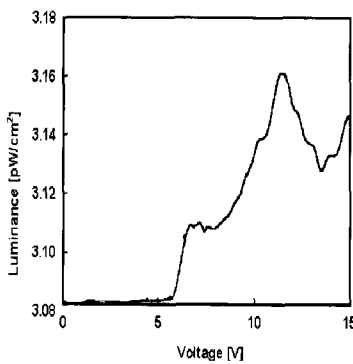
(b) 전압-휘도 특성
