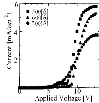
(a) 전압-전류 특성
