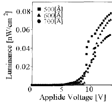
(b) 전압-휘도 특성
