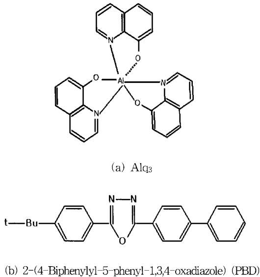
그림 1 분자 구조. Fig. 1 Molecular structure.
