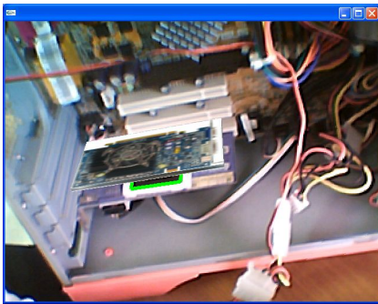
<그림 9> 그래픽카드 적용 실험
