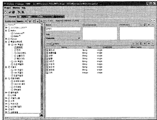
그림 3. protege-2000에서의 클래스 계층구조 Fig 3. class hierarchy on protege-2000
