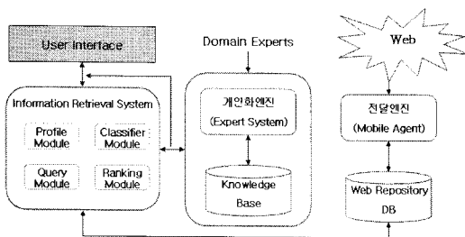
그림 6. 지능형 에이전트 시스템의 프로세스 Fig 6. process of intelligent agent system
