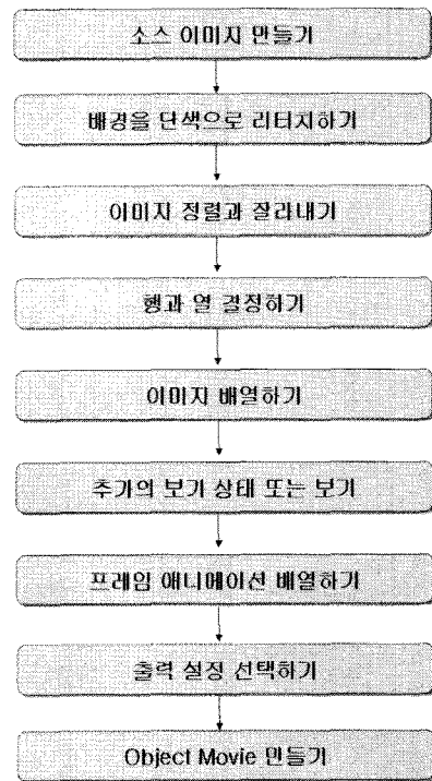
그림10 : QuickTime Mmovie 생성과정 Fig. 10. Process of QuickTime Mmovie Generation
