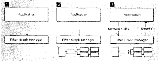
그림 6 어플리케이션, 필터그래프, 필터의 관계 Fig. 6. Application Filter v.s. Graph Filter
