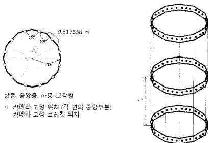
그림 8: 촬영 부스 설계도 Fig. 8. Design for Photographing Booth
