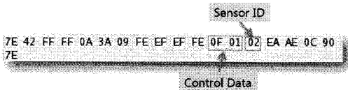
그림 11. 베이스 노드 전송 패킷 Fig. 11 Base Node Packet
