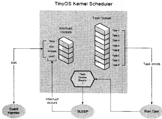
그림 8. TinyOS 커널 스케줄러 Fig. 8 TinyOS Kernel Scheduler
