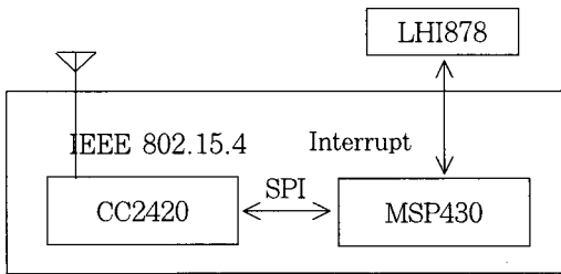
그림 5 센서노드부의 구성도 Fig. 5 Block Diagram of Sensor Node Part
