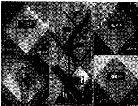
그림 12. 원격제어의 예 Fig. 12 Example of remote control
