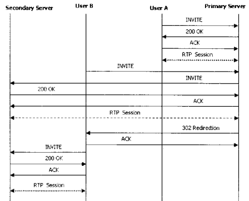
그림 3. 새로운 컨퍼런스 서버 추가 과정에서의 SIP 신호 처리 절차 Fig. 3. SIP Signaling Procedure while New Conference Server added
