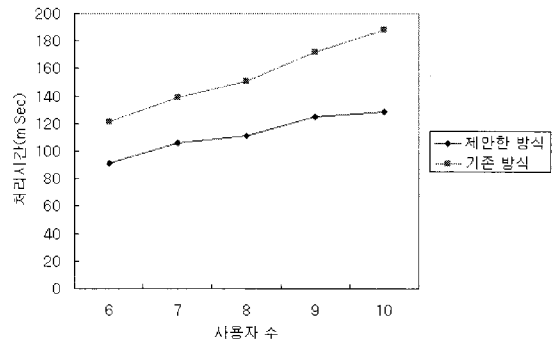
그림 5. 컨퍼런스 정보 통지 메시지 처리 시간 Fig. 5. Conference Notification Message Processing Time
