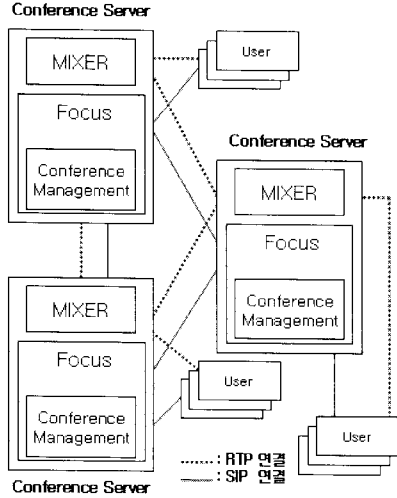
그림 2. 분산형 컨퍼런스 모델 Fig. 2. Distributed Conference Model
