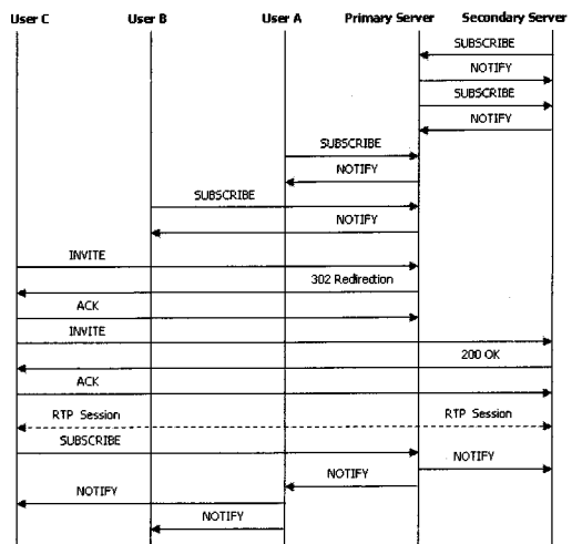
그림 4. 제안된 컨퍼런스 이벤트 패키지 동작 Fig. 4. Operation of Suggested Conference Event Package
