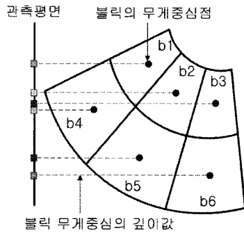
그림 6. 블럭들의 렌더링 순서를 정하기 위해 각 블럭 무게중심점의 깊이값을 비교 Fig. 6. Depth Value Calculation of Center of Gravity Points of the Bricks to Decide Rendering Order
