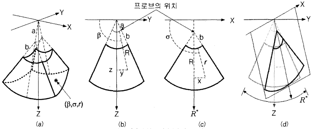
그림 3. 초음파 볼륨 데이터의 좌표 계산 Fig. 3. Coordinate Calculation of Ultrasound Volume Data
