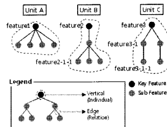
그림 2 피쳐간 결합도 Fig. 2 Coupling level between features
