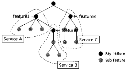
그림 4 독립성 측면의 정제 Fig. 4 Independency-side optimization
