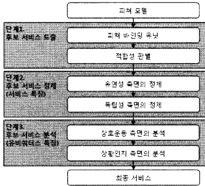
그림 1 피쳐 기반의 서비스 식별 프로세스 Fig. 1 Identification process of feature-based service
