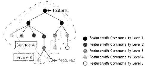
그림 3 유연성 측면의 정제 Fig. 3 Flexibility-side optimization
