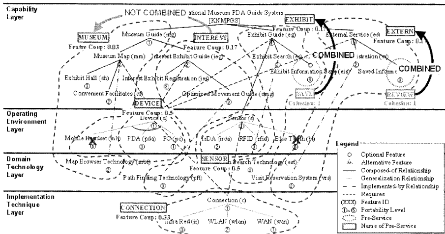
그림 7 KNMPGS에서 도출된 후보 서비스 Fig. 7 Drawn candidate-services of KNMPGS
