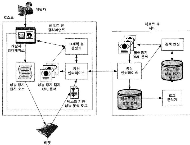
그림 2. 협업을 지원하는 임베디드 소프트웨어 성능 분석기의 전체 구성도 Fig. 2 Performance evaluation tool for embedded softwares on collaborative development environment
