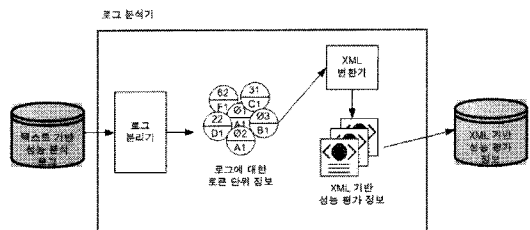
그림 3. XML 기반 성능 평가 정보 생성을 위한 로그 분석기 구성도 Fig. 3 Log separator for creating XML-based performance evaluation information
