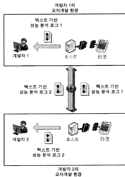
그림 1. 교차 개발 환경 Fig. 1 Cross development environment
