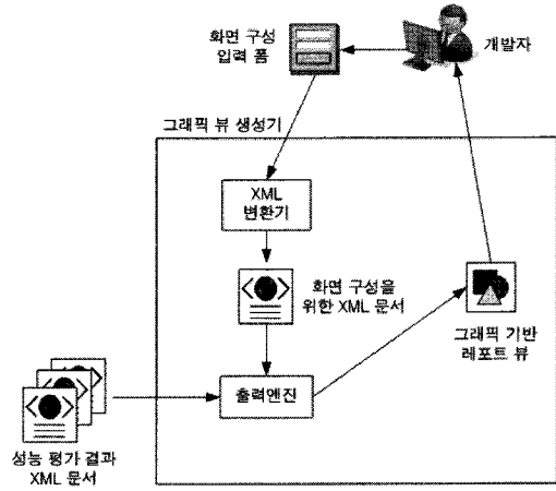
그림 5. 그래픽 뷰 생성기 구성도 Fig. 5 Graphic view generator
