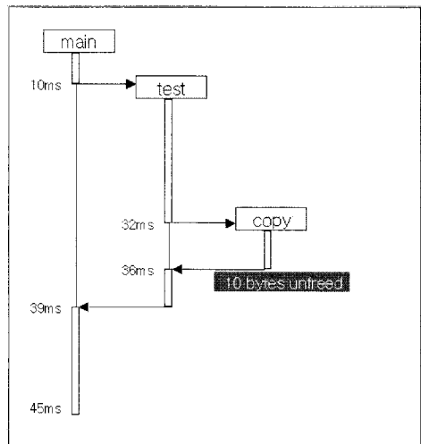
(a). 함수 관련 성능 분석 그래픽 뷰(시퀀스 다이어그램) (a). A graphic view for performance evaluation related in functions(Sequence diagram)
