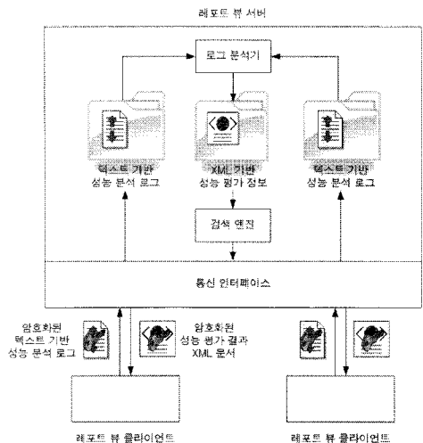
그림 4. 통신 및 문서 관리 메커니즘 Fig. 4 Mechanism for communication and document management
