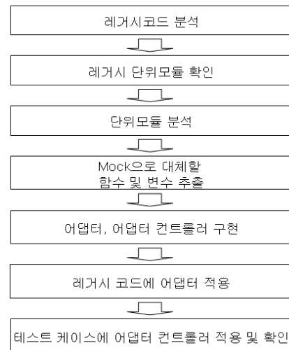
(그림 4) 레거시코드 재구성 흐름도
