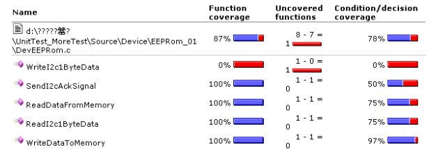
(그림 13) condition/decision 테스트 커버리지
