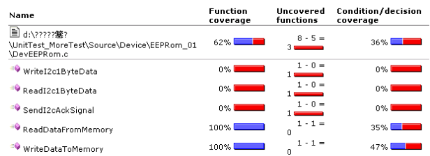
(그림 12) condition/decision 테스트 커버리지
