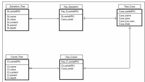
(그림 7) 데이터베이스의 구조
