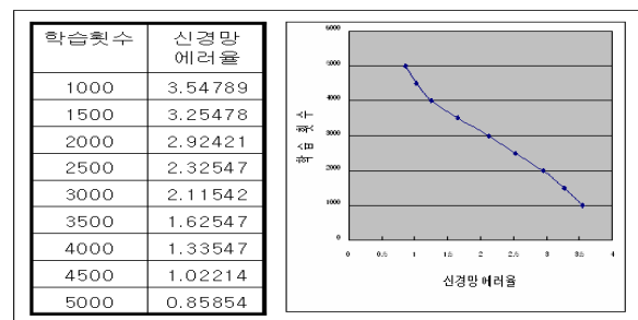
(그림 10) 신경망의 학습 횟수에 따른 에러율
