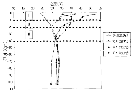
그림 11. 인천신공항 포장체 깊이별 온도분포의 시간에 따른 변화 예(1998년 8월 22일)
