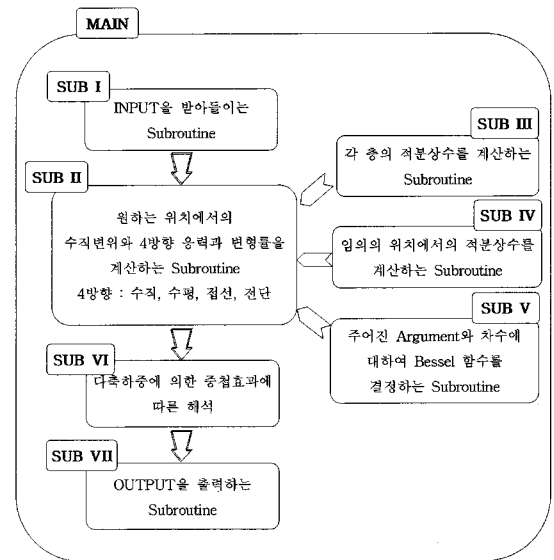
그림 1. 주프로그램과 부프로그램의 관계도
