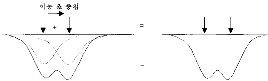
그림 2. 탄성해석에서 하중의 중첩효과
