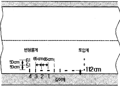
그림 13. 시험도로 계측기 매설위치의 평면도
