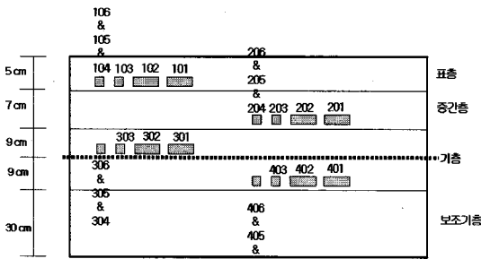
그림 14. 시험도로 계측기 매설위치의 단면도
