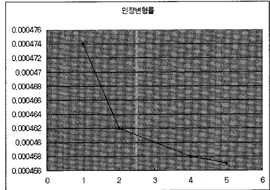
(a) 아스팔트층 하단의 인장변형률
