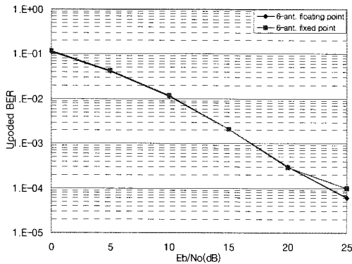
그림 7. 레일레이 페이딩 환경에서의 HSDPA 모드에서의 채널카드 성능
