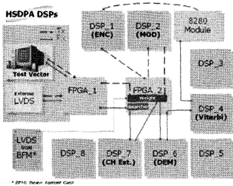
그림 4. HSDPA 모드에서의 DSP 할당
