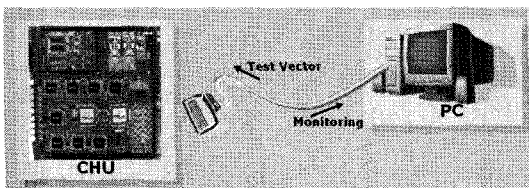
그림 5. PC와 채널 카드를 연결한 실험 환경
