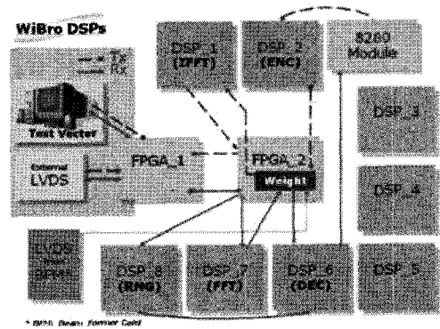
그림 3. WiBro 모드에서의 디바이스 할당
