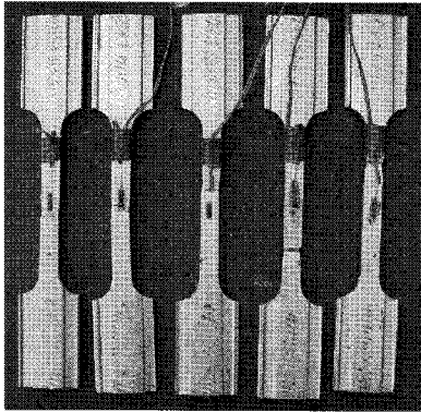
Fig. 3 Tensile Test Specimen.
