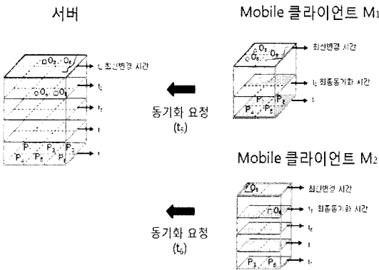
그림 1. 모바일 동기화요청의 예 Fig. 1 The example of mobile synchronization requests
