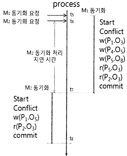
그림 2. M_1 과 M_2 의 동기화 예 Fig. 2 The example of serial synchronization for M_1 and M_2
