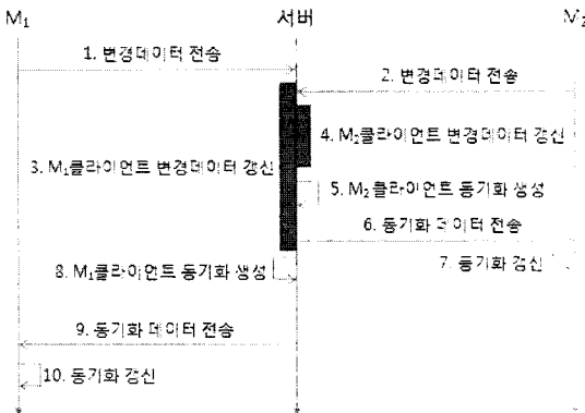
그림 3. 동시 동기화 프로토콜 Fig. 3 Concurrent synchronization protocol
