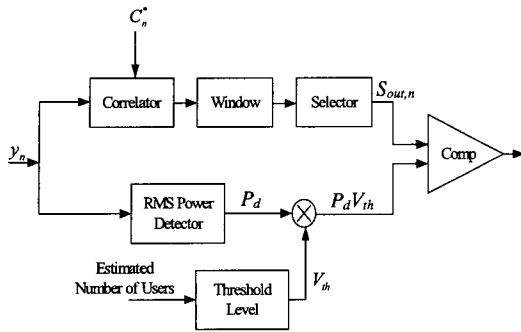
그림 2. GAS-CP-CDMA를 위한 초기 동기회로
