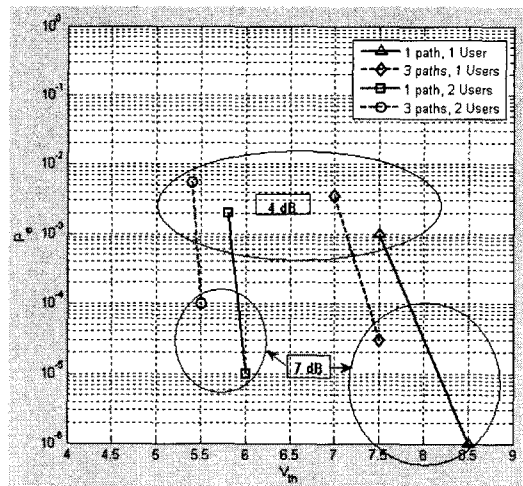
그림 6. 최적의 임계값에 따른 오류 확률 성능
