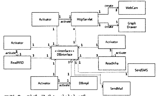
그림 3. 전체 클래스 다이어그램
