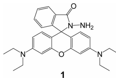
Scheme 1. Czamik's Cu 2+ -selective chemodosimeter 1 .
