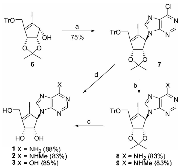
Scheme 3. (a) 6-chloropurine, \text{PPh}_3 , DEAD, THF, rt, 12 h; (b) \text{NH}_3/\text{MeOH} , 80^\circ\text{C} , 7 h for 8 ; 40% \text{CH}_3\text{NH}_2 , \text{MeOH} , 80^\circ\text{C} , 5 h for 9 ; (c) 2 N HCl, 1,4-dioxane, rt, 16 h for 1 and 2 ; (d) 1 N HCl, 1,4-dioxane, reflux, 15 h.
