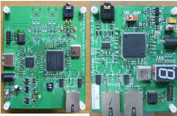
(그림 15) 보드 확대 사진(좌 : 전송부, 우 : 수신부) (Fig. 15) Board enlargement photographs (left : transmission part, right : receiving part)
