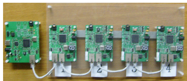
(그림 14) 전송부와 수신부를 연결한 사진 (Fig. 14) Photograph for transmission and receiving connection
