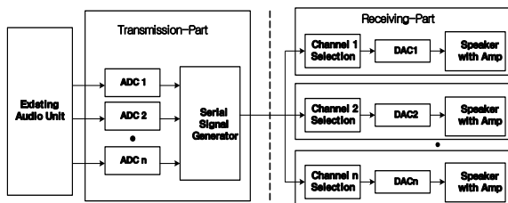
(그림 1) 기존 전송 및 수신측 블록도 (Fig. 1) Transmission and Receiving-part block diagram of the existing system
