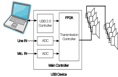
(그림 2) USB 인터페이스 스피커의 직렬연결 방법 (Fig. 2) Serial connection method of speakers by a USB interface
