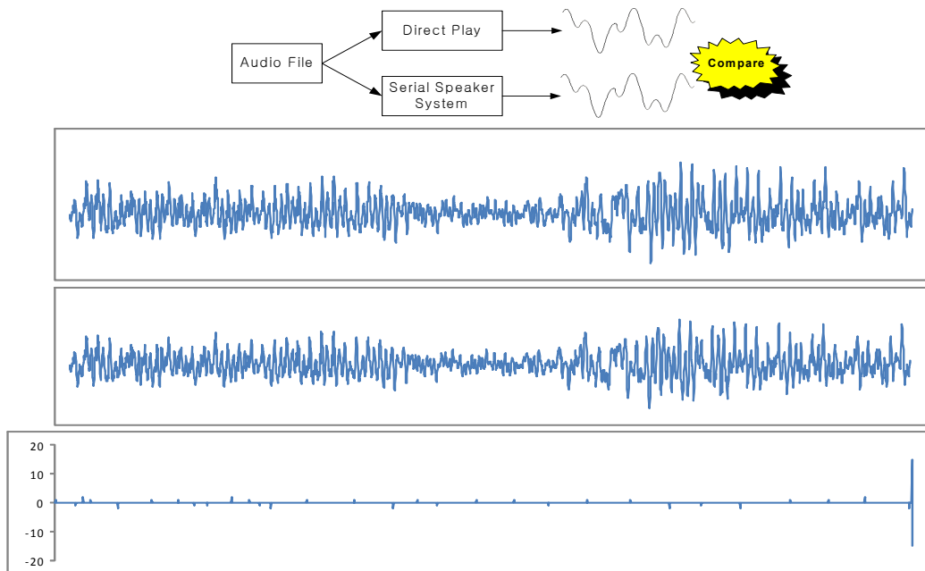
(그림 16) 원래의 오디오 신호와 재생 신호의 파형 비교 (Fig. 16) Waveform comparison of original signal and and regenerated signal
