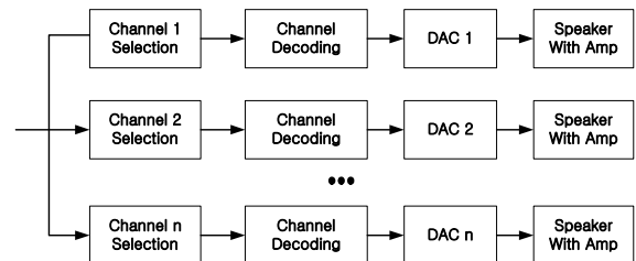
(그림 7) 수신측 블록도 (Fig. 7) Receiving part block diagram
